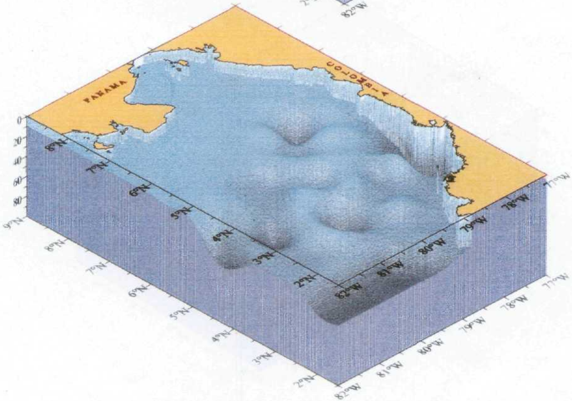
Figura 2: Distribución del promedio mensual de profundidad de la termoclina en Enero y Marzo en la Cuenca del Pacifico Colombiano
