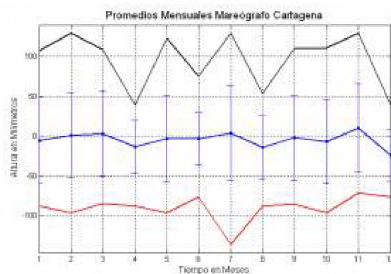
Figura 5. Promedios mensuales de 41 años de datos horarios del mareógrafo de Cartagena.
