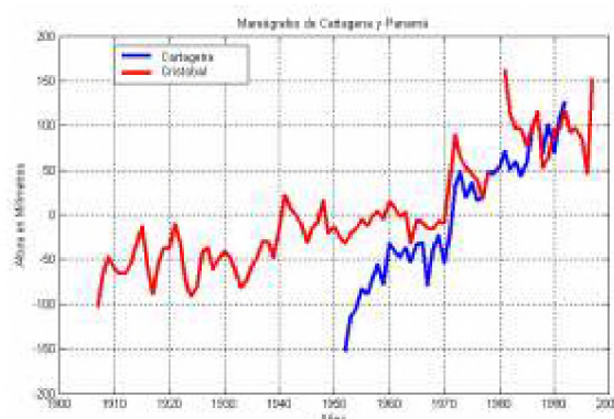
Figura 4. Series de Tiempo de nivel del mar en Cartagena y Cristóbal. Promedios anuales con base en datos horarios, restando el promedio multianual.
