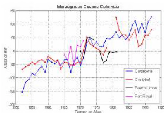
Figura 3. Series de Tiempo de nivel del mar en Cartagena, Cristóbal, Puerto Limón y Port Royal. Promedios anuales con base en datos horarios, restando el promedio multianual.
