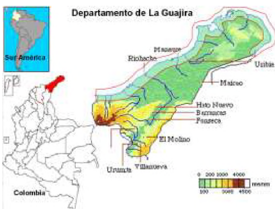
Figura 1. Esquema de localización del Departamento de La Guajira en la península nordeste que lleva su nombre en el norte de Colombia, esquina noroccidental de América del Sur. La zona resaltada en transparencia azul y bordes rojos, corresponde a la zona costera del área de estudio, entre el Municipio de Palomino, al oeste y El Hito Internacional Castilletes al nordeste.
