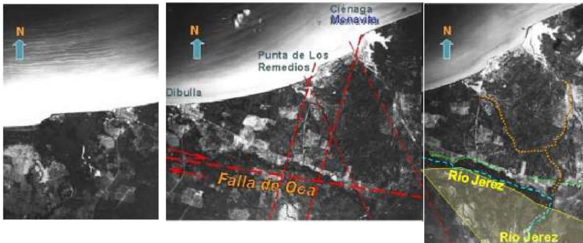
Figura 4. Tripleta estereográfica no a escala del sector entre Punta El Sequión (al Oeste de Dibulla) y Ciénaga Monavita (al Este de Punta de Los Remedios). Se resalta el trazo aproximado de la Falla de Oca, la cual controla el curso del Río Jerez (azul); y los lineamientos asociados en sentido SW-NE y SE-NW. El Río ha disectado el abanico-terracea y ha formado escarpes (líneas verdes) al borde de conos-terracea. A lo largo del valle, aún se diferencian entre dos y tres niveles de terrazas, así como facetas triangulares. Nótese en línea punteada anaranjada, antiguos cauces del río entre depósitos distales, a su vez afectados por dichos lineamientos.
