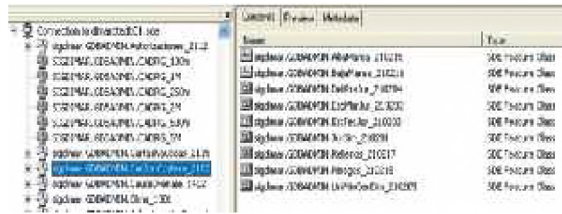
Figura 14. Feature Class presentes en el Feature Dataset de zona costera en la Geodatabase Corporativa de la DIMAR.
