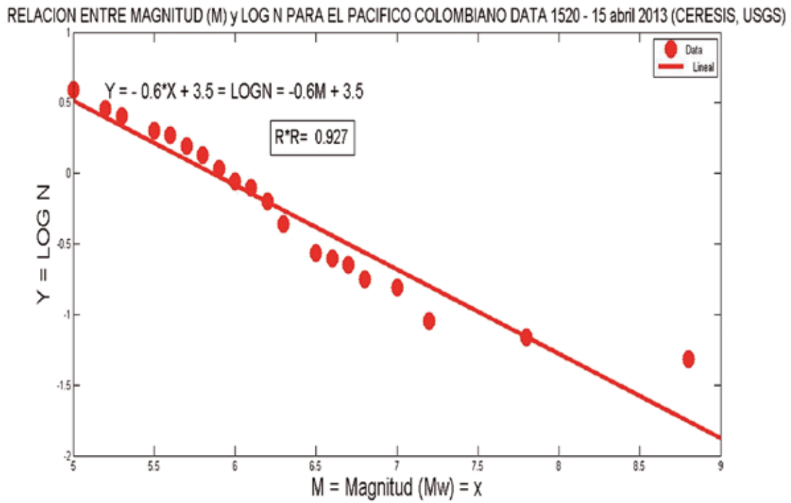
Figura 6. Relación entre magnitud y LOGN para el Pacífico colombiano, data (1520-15 abril 2013 Ceresis, USGS) latitud 0° a 7.5°.
